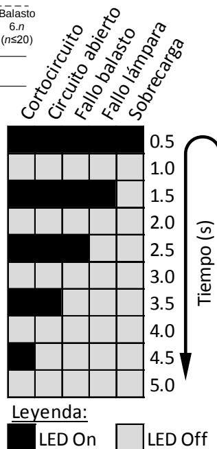
Figura 2. Notificación de errores de LED de estado de canal DALI
