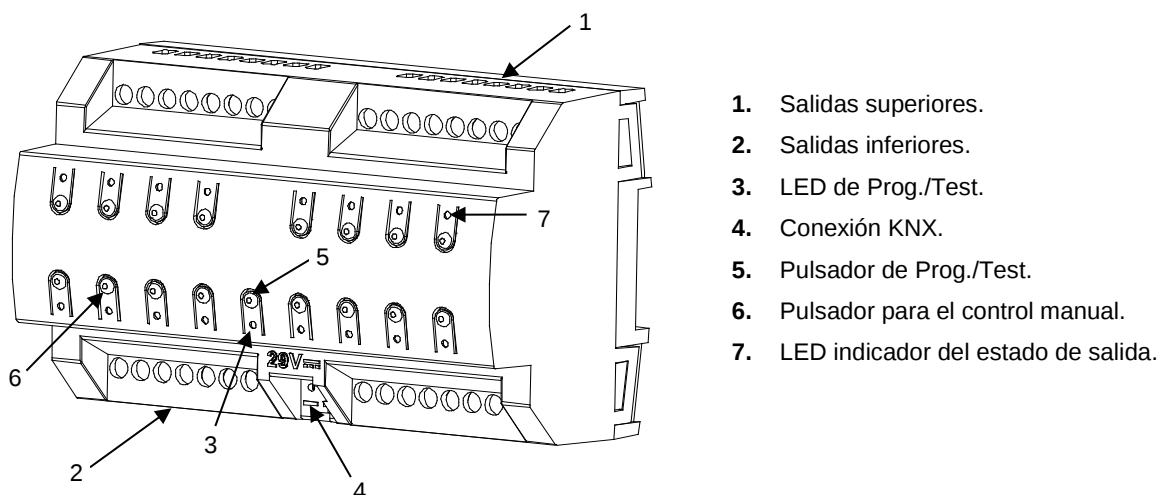
Figura 1 MAXinBOX FANCOIL 4CH2P. Elementos.
