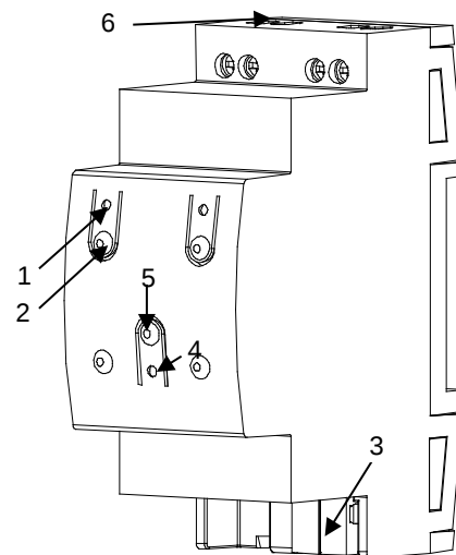
Figura 1. MINiBOX 20
