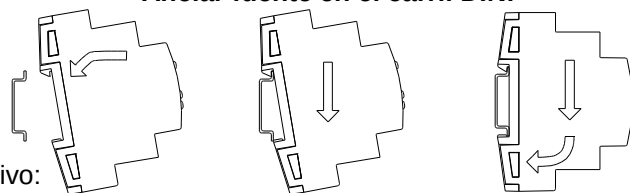
Figura 2: Instalación y conexión ZPS320HIC230
