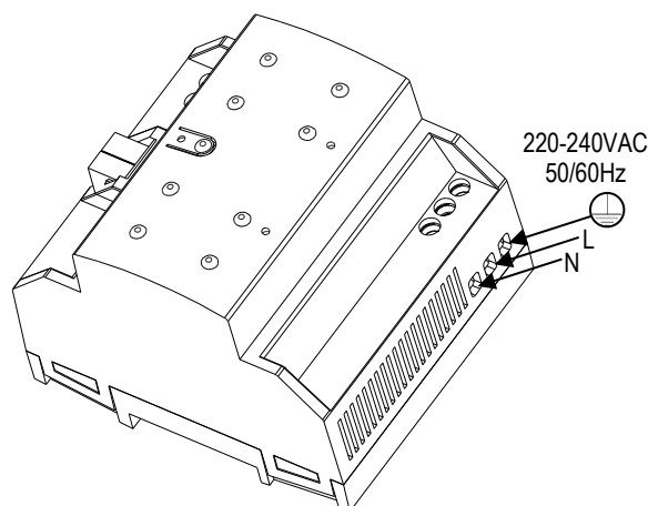
Figura 2: Instalación y conexión ZPS320HIC230
