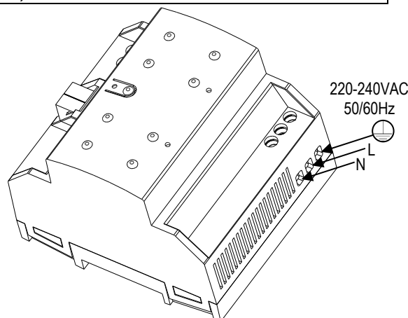
Figura 2: Instalación y conexión ZPS640HIC230
