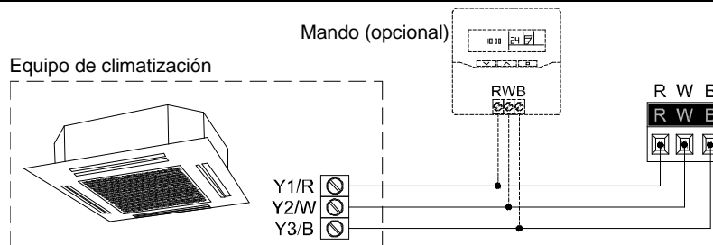
Figura 2. Cableado de KLIC-FJ al equipo de climatización
