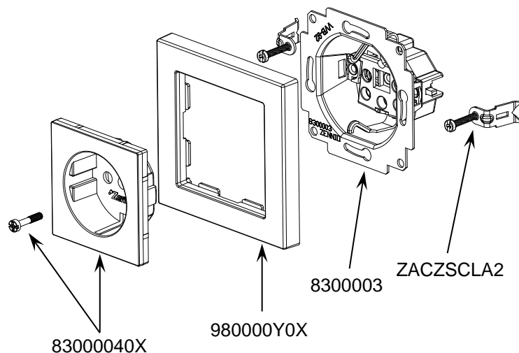
Figura 1. Toma de enchufe Schuko.
