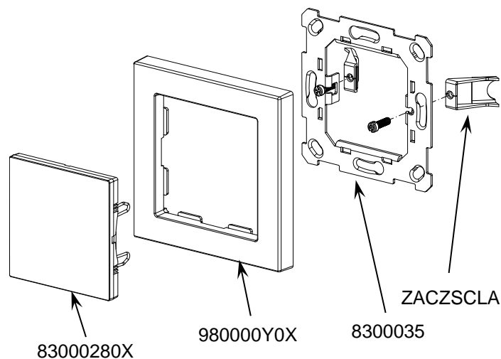
Figura 1. Tapa ciega.
